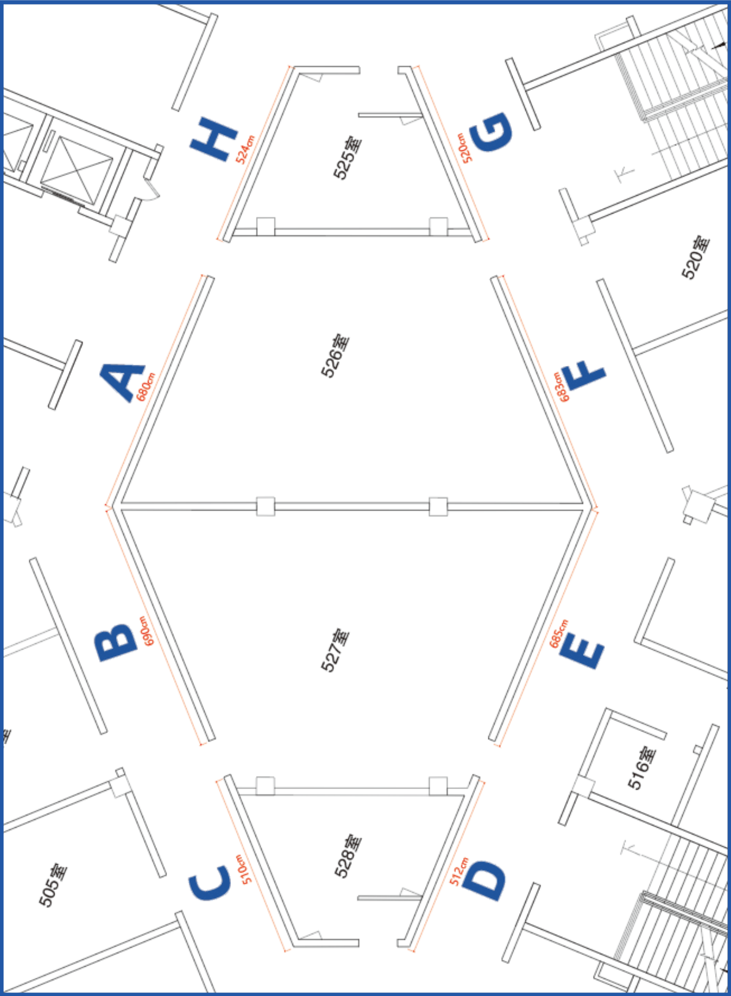
五楼平面图：
